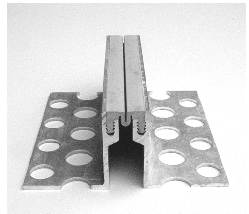
perfil BF 15
