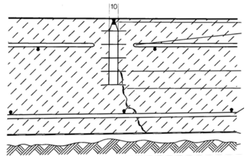
perfil SF 80
